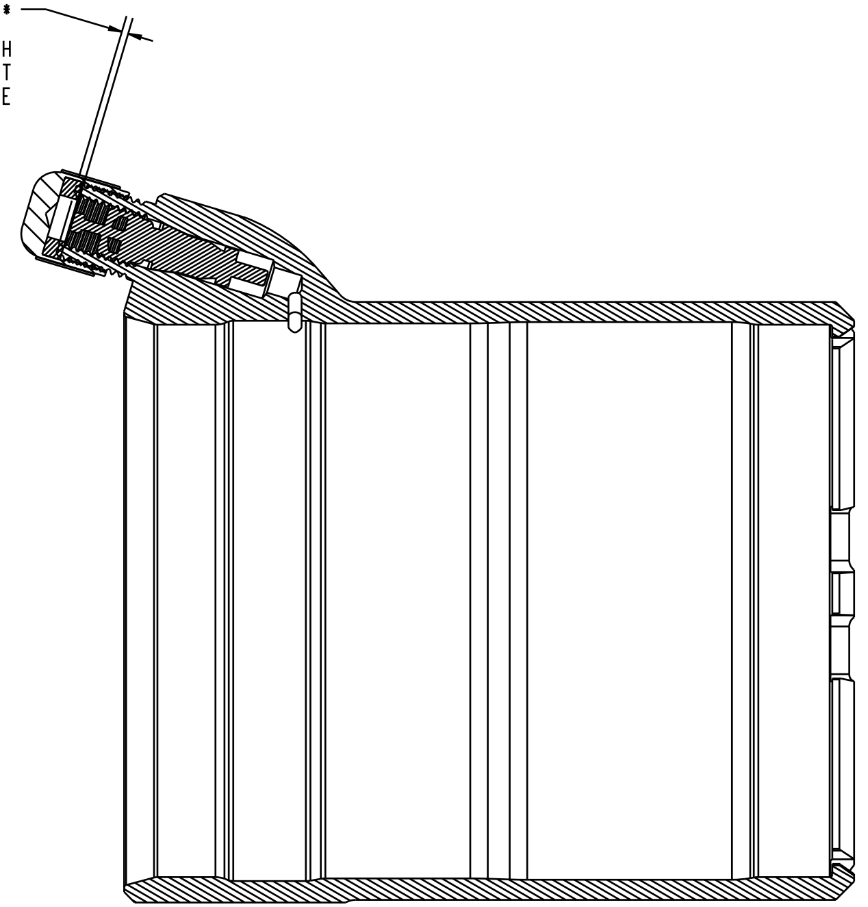
SECTION A-A
